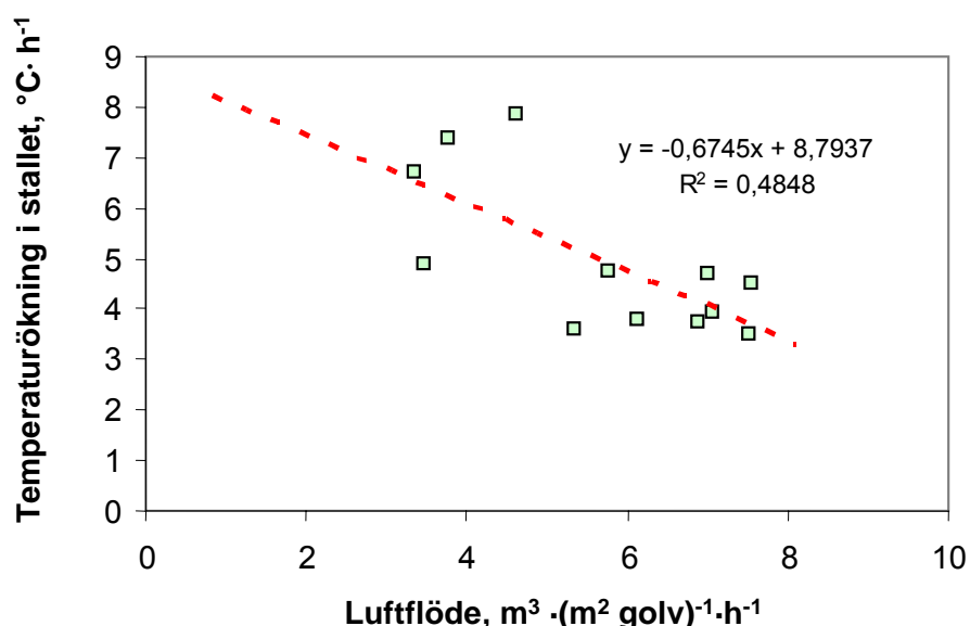
Figur 38. Temperaturökningshastighet i byggnad 1 under ca 30 minuters (medel 33 min) tillförsel av värme med effekten 55 \text{ W/m}^2 golvyta. Medeltemperatur utomhus 22,9 \text{ }^{\circ}\text{C} . Medeltemperaturskillnad 3,7 \text{ }^{\circ}\text{C} mellan stallluft och utomhusluft vid start.
