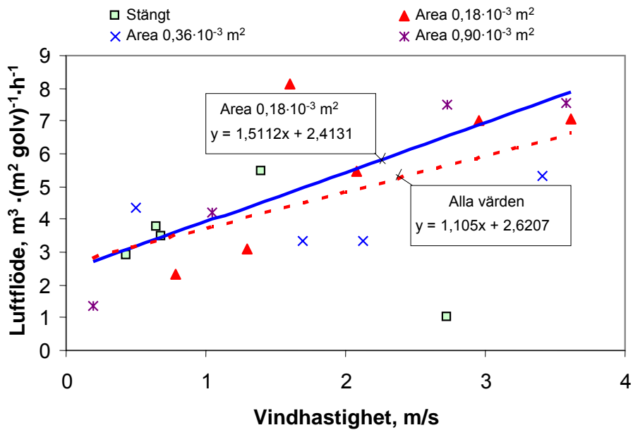
Figur 30. Inverkan av vindhastighet på ventilationsflöde i byggnad nr 1 vid stängda spaltdon och öppet frånluftspjäll.
