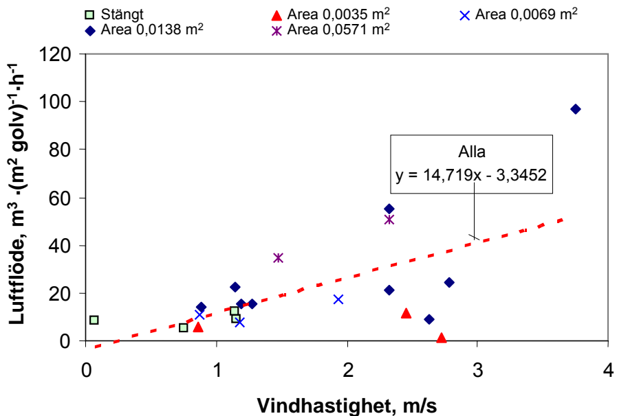
Figur 31. Inverkan av vindhastighet på ventilationsflöde i byggnad nr 3 vid öppna sidoluckor och stängd taknock.
