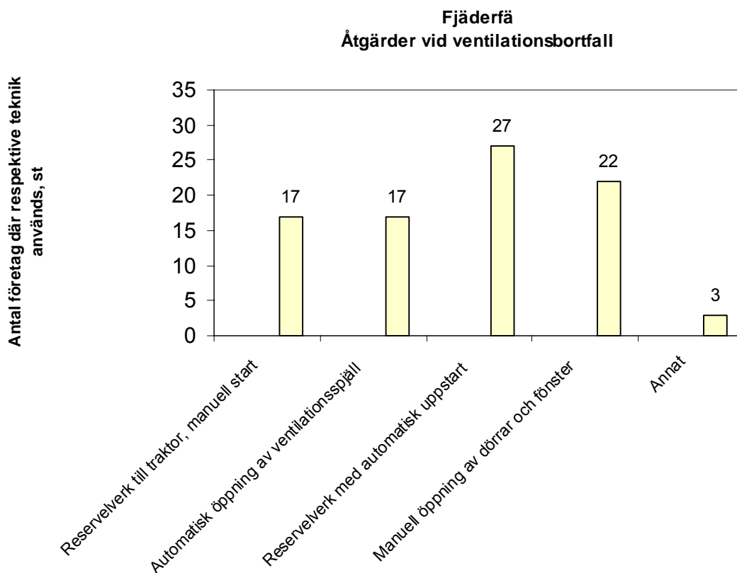
Figur 16. Åtgärder för nödventilation vid ventilationsbortfall på gårdarna med fjäderfä.
