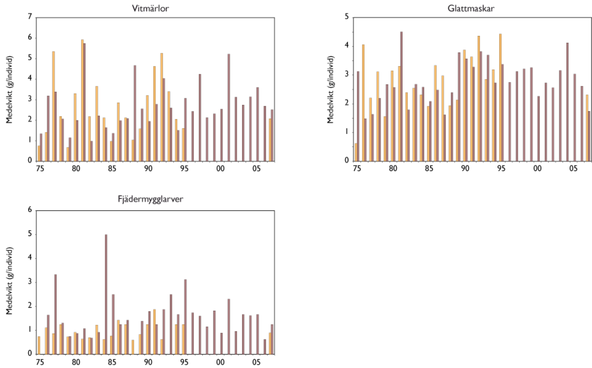
Figur 3. Medelvikten vid vår- och höstprovtagningar (maj resp. augusti) för vitmärlor, glattmaskar och fjädermygglarver vid Tärnan 1975-2007.
