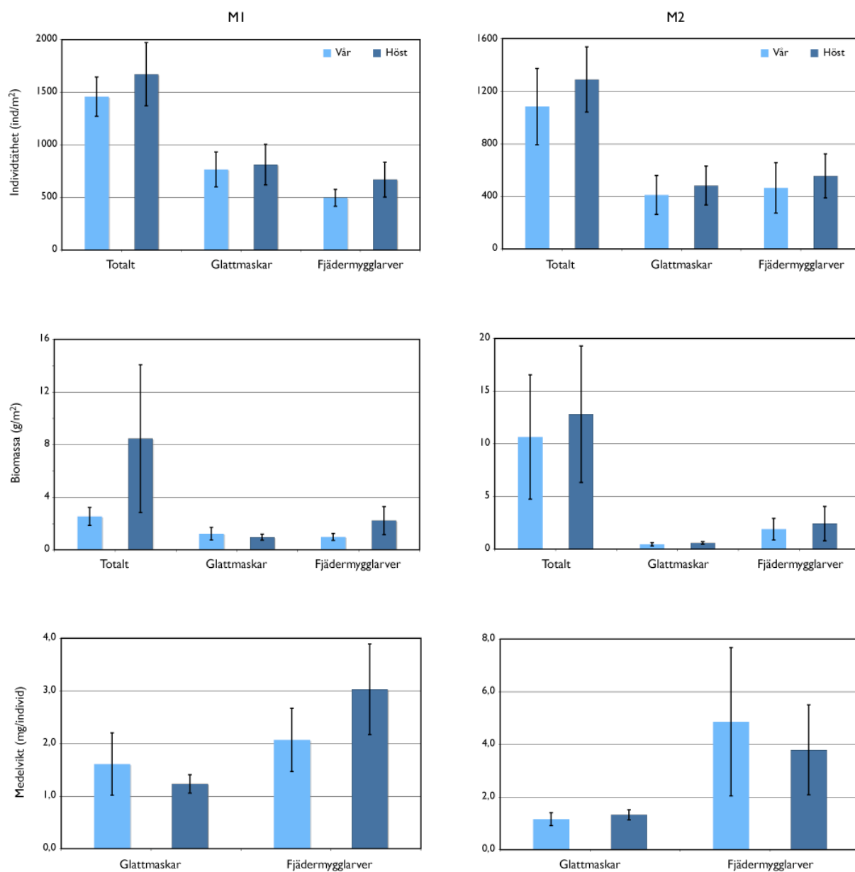
Figur 6. Medelvärden och 95%-iga konfidensintervall för individtheter, biomassa och medelvikt för vår- och höstprovtagningar vid provplatserna M1 och M2 i Mariestadsfjärden 1984–2006.
