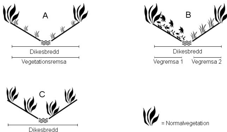
Figur 6.6. Schematisk bild över koppling av dike till vegetationsremсор. A) Överlappande, B) Anslutande, C) Friliggande.
