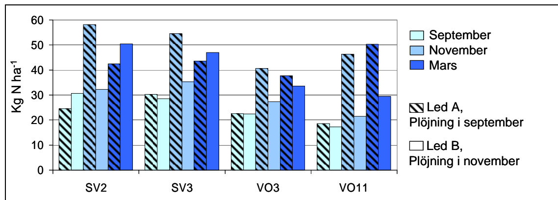
Figur 8. Mineralkväve ( \text{NH}_4^+ och \text{NO}_3^- ) ( \text{kg N ha}^{-1} ) i markprofilen (0-90 cm) i fyra försök vid tre provtagningstillfällen (september och november 2002 samt mars 2003).
