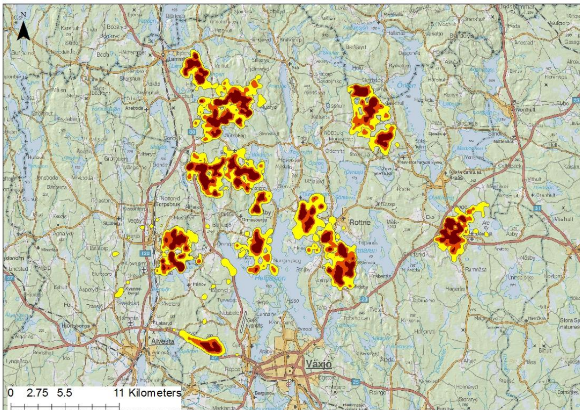
Figur 3. Årshemområden för 21 GPS-märkta älgkor i Växjöområdet under 2016/2017. Områden de rör sig över under hela året (gul, 95 % skattningar) och kärnområden (röd, 50 % skattningar).
