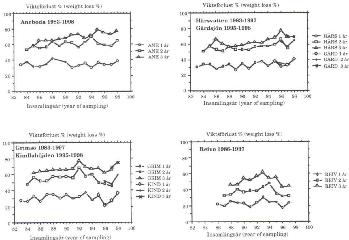
Figur 3. Tidsserier för nedbrytning av ett-, två- och treårig standardförna (tallbarr) från fyra lokaler. Viktsförlusten angiven i procent av torrsvikt vid start. Time series for decomposition of one, two and three years old standardised litter (pine needles) at four sites. Weight loss expressed as percentage of initial dry weight.
