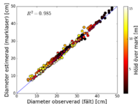
Figur 3. Detektering av stamprofiler med terrester laserskanning är fullt jämförbar med manuell fältmätning. Upp till femton meter över marken hittas de flesta stamdiametrar och de automatiska mätningarna ligger väldigt nära de manuellt framtagna (RMSE = 11 mm).
