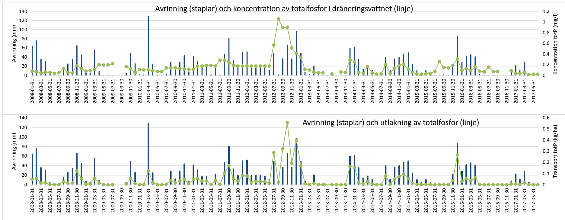
Figur 17 a-b. Månadsdynamik hos avrinning och koncentrationer av totalfosfor och den beräknade fosfortlakningen i Lannaförsöket 2008-2017.
