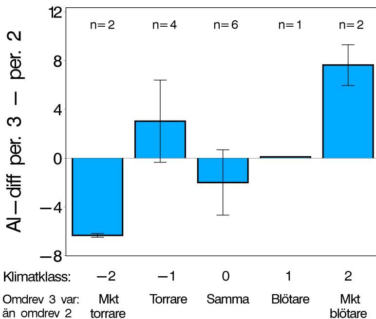
Figur 7. Förändringen av utbytbart Al (mmolc/kg torrs substans) i B-horisonten mellan inventeringsperioderna 1993-2002 och 2003-2012 uppdelat på de nya klimatklasserna. Signifikanta skillnader i förändringen av utbytbart Al mellan klimatklasserna -2 och 2.
