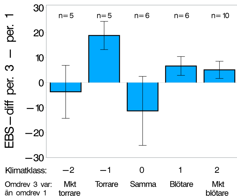
Figur 5. Förändringen av effektiv basmättnadsgrad (i %) i O-horizonten mellan inventeringsperioderna 1983-1987 och 2003-2012 uppdelat på de nya klimatklasserna. De blå staplarna visar medelvärdet av förändringen i effektiv basmättnadsgrad inom respektive klimatklass och felstaplarna visar medelfelet. Signifikant skillnad i förändringen av effektiv basmättnadsgrad mellan klimatklasserna -1 och 0.
