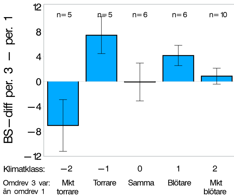
Figur 4. Förändringen av basmättnadsgraden (i %) i O-horizonten mellan inventeringsperioderna 1983-1987 och 2003-2012 uppdelat på de nya klimatklasserna. De blå staplarna visar medelvärdet av förändringen i basmättnadsgrad inom respektive klimatklass och felstaplarna visar medelfelet. Signifikanta skillnader i förändringen av basmättnadsgraden mellan klimatklasserna -2 och -1, -2 och 1, samt mellan -2 och 2.
