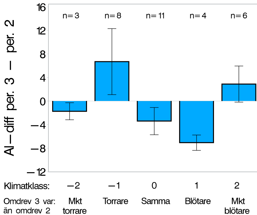
Figur 6. Förändringen av utbytbart Al (mmolc/kg torrs substans) i O-horisonten mellan inventeringsperioderna 1993-2002 och 2003-2012 uppdelat på de nya klimatklasserna. Signifikanta skillnader i förändringen av utbytbart Al mellan klimatklasserna -1 och 0, samt mellan -1 och 1.
