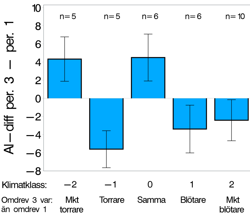
Figur 3. Förändringen av utbytbart Al (mmolc/kg torrsbstans) i O-horisonten mellan inventeringsperioderna 1983-1987 och 2003-2012 uppdelat på de nya klimatklasserna. De blå staplarna visar medelvärdet av förändringen i utbytbart Al inom respektive klimatklass och felstaplarna visar medelfelet. Signifikanta skillnader i förändringen av utbytbart Al mellan klimatklasserna -2 och -1, -1 och 0, 0 och 2, samt mellan 0 och 1.
