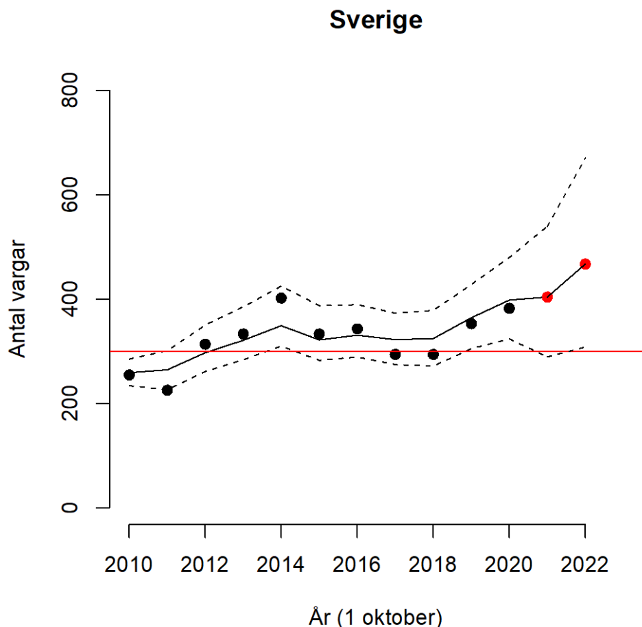
Figur 3. Populationsstorlek (beräknat som antal för yngningar \times 9,8 ) i relation till år (1 oktober, d.v.s. vid inventeringsperiodens start, svarta punkter). Prognoser (röda punkter) för 1 oktober 2021 (med beskattning på 49 vargar under perioden 1 oktober 2020 – 30 april 2021), samt för 1 oktober 2022 (utan någon jakt). Modellprediktion (linje och 90 % KI; streckade linjer). Nivån för gynnsam bevarande status (300 vargar, röd horisontell linje). Under perioden var median tillväxttakten ( \lambda ) = 1,16 (0,98 – 1,35, 90% KI).
