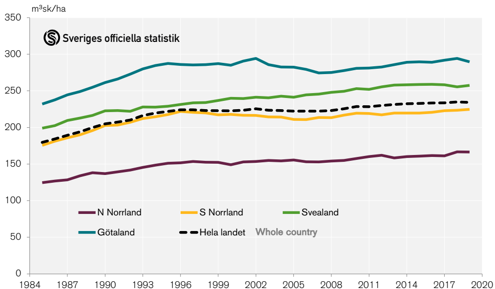
Figur 3.20 Virkesförråd levade träd per hektar i skog som har uppnått rekommenderad ålder för föryngringsavverkning. 1985–2019.
