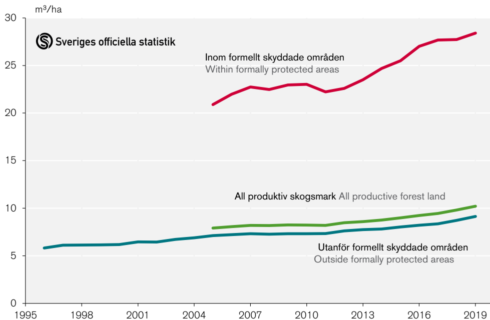
Figur 3.27 Volym död ved per hektar inom och utom formellt skyddade områden. 1996–2019.
