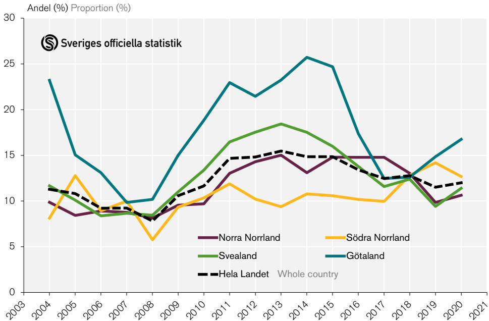
Figur 3.34 Andel tallstammar med färsk skada av älgbetningsskador. 2004–2020.
