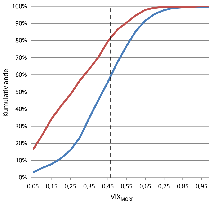
Figur 19. Den kumulativa andelen av totalantalet (%) av opåverkade (blå) och påverkade (röd) mot VIX_{MORF} . Påverkade består av påverkanstrycken rensning och kanalisering i klasserna 2 och 3 och opåverkade är bedömda som utan påverkanstryck. Den lodräta linjen visar brytpunkten mellan påverkade och opåverkade lokaler ( VIX_{MORF} 0,467).
