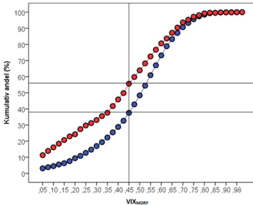
Figur 16. Den kumulativa andelen av totalantalet (%) opåverkade (blå) och påverkade lokaler (röd) i förhållande till VIX_{MORF} . Den lodräta linjen visar ett exempel på en brytpunkt mellan påverkade och opåverkade lokaler på 0,45 och de vågräta linjerna visar effekten på andelen opåverkade och påverkade lokaler.
