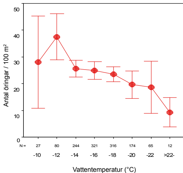
Figur 3. Tätheten av örting (beräknat antal individer per 100 m² vattendragsyta) på de lokaler där arten förekom avsatt mot vattentemperaturen vid elfisket i augusti. Avser endast inlandsvattendrag söder om Dalälven (Halldén & Degerman 2003). Medelvärde plus/minus 95 %-konfidensintervall angivet.
