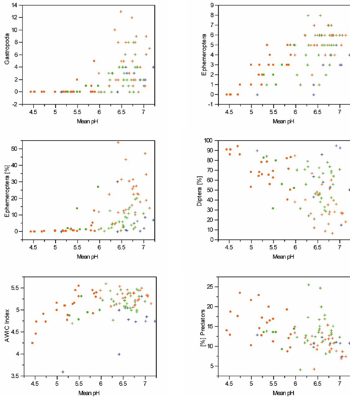
Figur 16. Diagram för de sex indexen som ingår i MILA indexet längs en pH gradient (medel pH). Blå = Boreala höglandet, grön = Fennoskandiska skölden och röd = Centralslätten. Kryss = referenser. Gastropoda = snäckor, Ephemeroptera = dagsländor, Diptera = tvåvingar, AWIC hänvisar till ett engelskt försurningsindex (se text).
