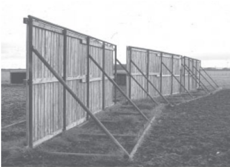
Figur B 6:2. Exempel på kanadensiskt flyttbart vindsyddsstaket. Normalt är vindsyddsstaket permanenta.
