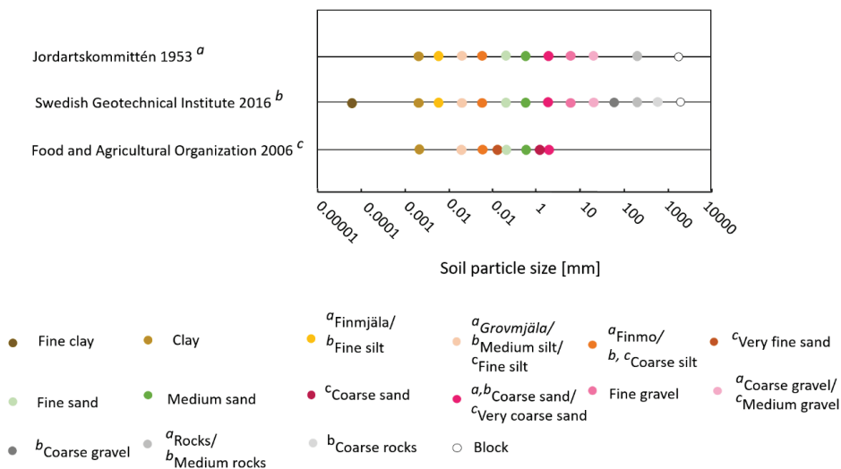
Figure S 1 Differences in classification of soil particle size between major soil classifications systems in Sweden (Atterberg's grain size intervals) (Jordartskommittén (1953). Jordartsnomenklatur utarbetad av representanter för Kongl. Skogshögskolan, Statens Geotekniska Institut, Statens Väginstitut och Sveriges Geologiska Undersökning I juni 1953, Opublicerat protokoll) (a), Swedish Geotechnical Institute (SGI) (Karlsson, C., Sohlenius, G. & Becher, G.P. (2021). Handledning för jordartsgeologiska kartor och databaser över Sverige. SGU-rapport 2021:17. Geological Survey of Sweden.' (b)) and international (Food and Agricultural Organization (2006). Guidelines for soil description. 4th ed. Rome: Food and Agriculture Organization of the United Nations. https://www.fao.org/3/a0541e/a0541e.pdf , (c))
