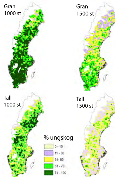
Figur 3. Rumslig fördelning av gran- och talldominerade ungskogar i Sverige med mer än 1000 stammar per hektar (till vänster) och 1500 stammar per hektar (till höger).
