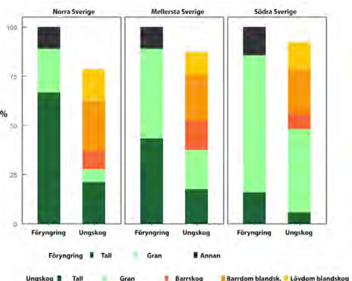
Figur 4. Trädslagssammansättning dels i förnygringarna, dels i ungskogarna. Andel (%) av arealen.
