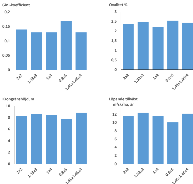
Figur 4. Exempel på några egenskaper i tallförsöket i Siljansfors vid 37 års ålder i försöksleden med olika planteringsförband: Ginikoefficient, ovalitet, krongräns höjd och löpande tillväxt. Inga av skillnaderna var signifikanta.
