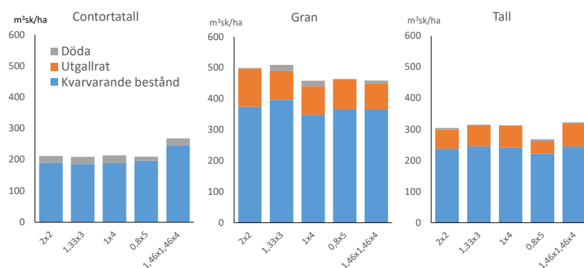
Figur 3. Total volymproduktion vid mätningar 2016 (gran) och 2020 (contortatall och tall).
