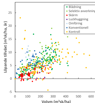
Figur 3. Löpande tillväxt i förhållande till stående volym för provtytor i hyggesfria försök. "Konventionell" är trakthyggesbruk och "kontroll" är obehandlade provtytor (fri utveckling).
