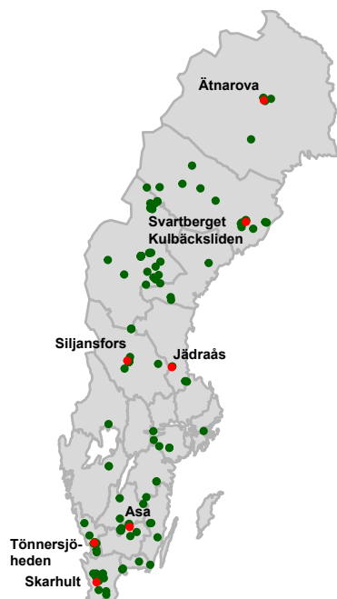
Figur 2. Lokalisering av långsiktiga fältförsök kopplade till hyggesfritt skogsbruk (grön) och försöksparkerna (röd). Vissa försök ligger på samma lokal, vilket gör att punkterna överlappar varandra.
