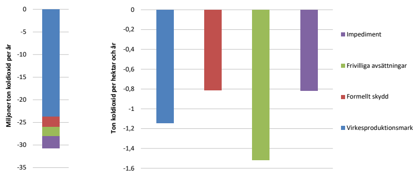
Figur 6. Nettoppdrag i biomassa på skogsmarkskategorier 2016. Totalt per kategori (vänster) och per hektar (höger).
