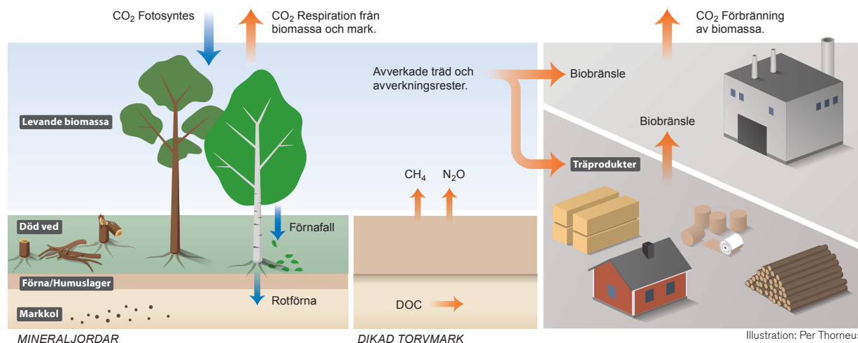
Figur 2. Figuren visar kolets kretslopp i förhållande till de kolpooler (vit text med grå bakgrund) som redovisas i klimatrapporteringen. Kolförrådsförändringar som rapporteras representerar skillnaden mellan inflödet och utflödet av kol för en kolpool. För kolpoolen levande biomassa representerar kolförrådsförändringen skillnaden mellan upptag genom fotosyntes och utsläpp på grund av respiration, avverkning och naturlig avgång.
