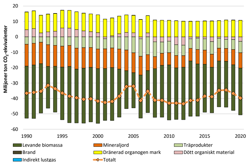
Figur 5. Nettoppdrag (negativa värden) och nettoutsläpp (positiva värden) fördelat på kolpooler, träprodukter (HWP) och andra utsläpp. Källa: www.naturvardsverket.se
