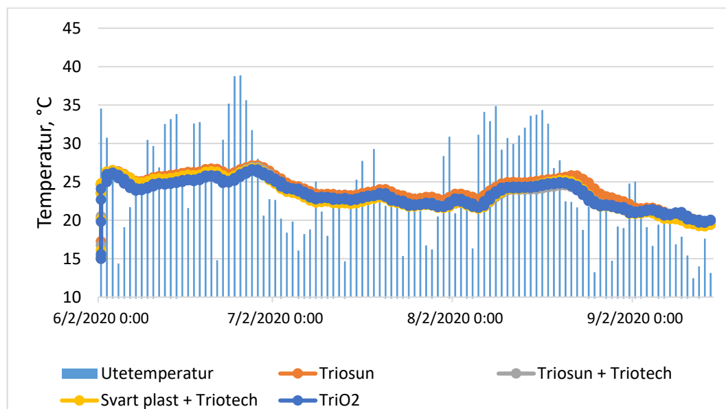
Figur 2. Temperatur i ensilage lagrat i plansilo täckt med olika plastfilmer (linje) och utetemperatur (stapel) 2020.
