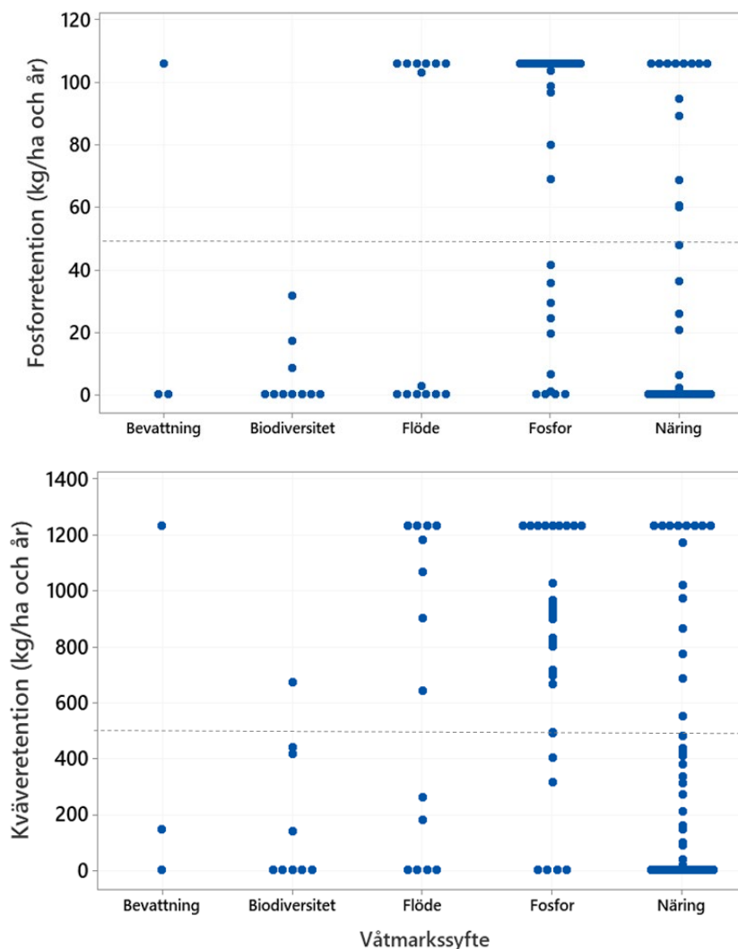
Figur 8. Kväve- och fosforretention i de våtmarker och dammar som anlagts med LOVA-stöd 2017-2021. Våtmarkernas huvudsyfte var näringsrening eller biologisk mångfald och dammarna anlades för bevattning fosfor eller flödesdämpning.
