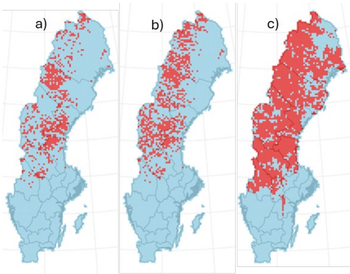
Figur 13. Områden i Sverige där olika alternativ uppfyllts per ruta om 10 × 10 km (markerade i rött): a) spårning minst 1 km eller tills DNA-prov hittats, b) minst ett ID-bestämt prov och c) sökinsats om minst 20 km.
