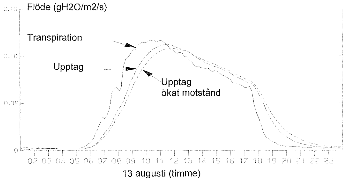
Figur 4.7. Simulerad transpiration och upptag. Dels för ett standard fall, dels för ett fall då växtmotståndet ökats med knappt 40%. Samma växt, mark och väder förhållanden, samt modell som i figur 4.2.
