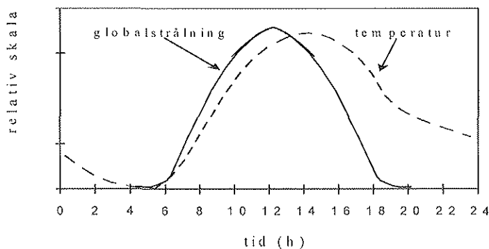
Figur 8.2. Relativ solinstrålning och lufttemperatur ovan bar mark (omritad efter Rosenberg et al, 1983)
