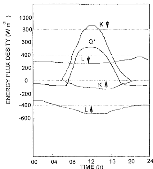
Fig.7.4. Komponenter i strålningsbalansen den 30 juli i Matador, Saskatchewan ( 50^{\circ}\text{N} ) över ett bestånd av 0,2 m präriegräs. Molnfri himmel på morgonen, ökande molnighet sent på eftermiddagen och kvällen. Observera att inkommande strålning till ytan är ritade som positiva och utgående strålning är ritad med negativa värden. (Efter Ripley and Redman, 1976)
