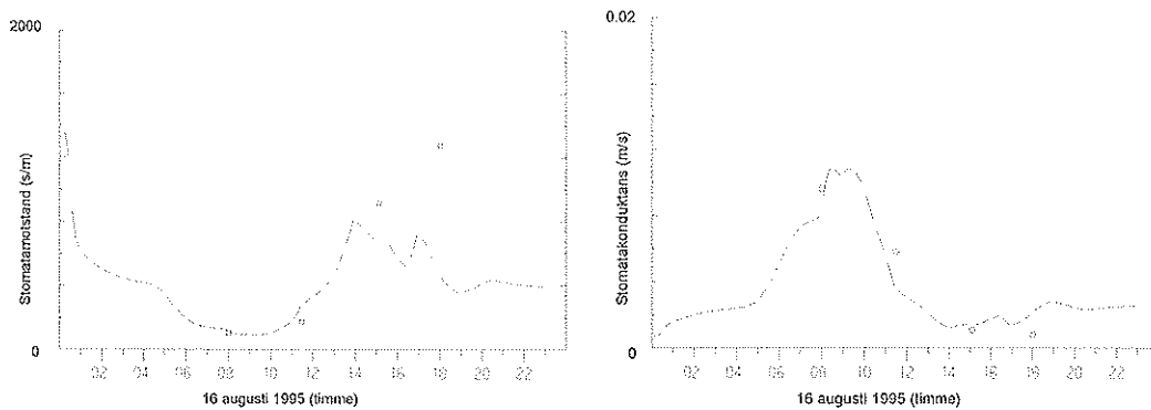
Figur 5.8a och b. a) Stomatarmotståndet ( r_c , i ekv 4.3) hos unga granplantor i Östad (Västergötland) simulerat (linje; SPAC-modellen) som funktion av infallande strålning, ångtrycksdeficit samt markens och barrens vattenpotential. Mätningarna (punkterna) och drivdata till simuleringarna är gjorda av Per-Erik Karlsson, Institutet för Vatten och Luftvårdsforskning (IVL, Göteborg). b) Stomatakonduktansen beräknad som inversen av värdena i figur a.
