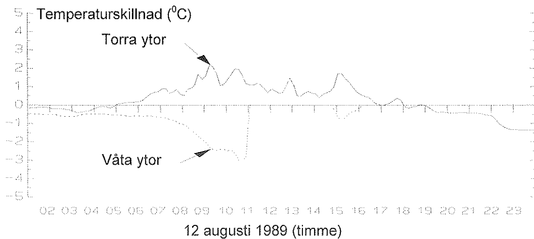
Figur 4.10. Skillnaden mellan bladens temperatur och luftens temperatur en regnig sommardag, dels för de transpirerande ytorna dels för de våta ytorna med interceperat vatten (samma förutsättningar som i figur 4.9).
