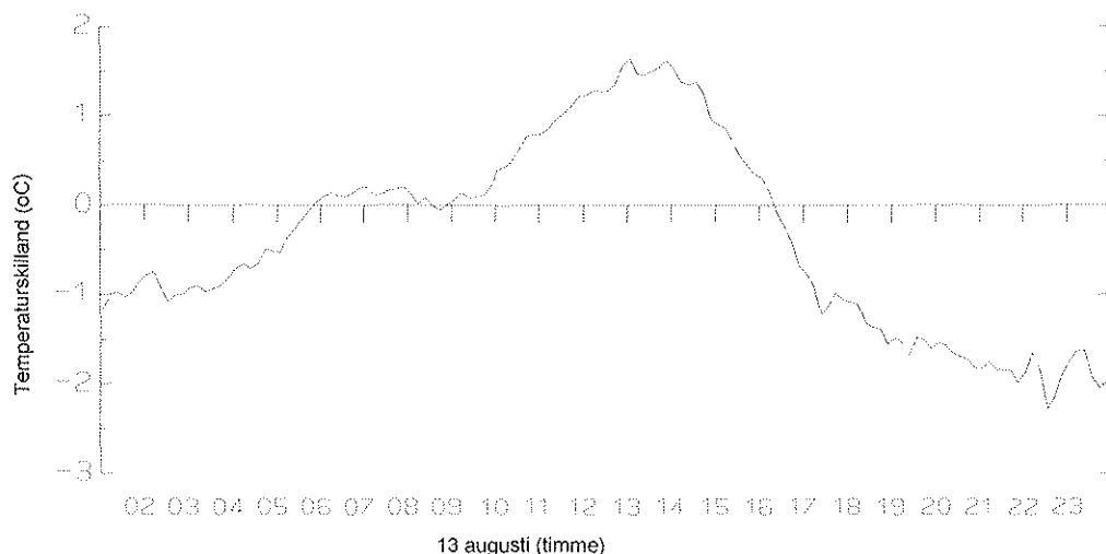
Figur 4.3. Skillnaden mellan bladens temperatur och luftens temperatur en solig sommardag simulerad med SPAC. Samma växt, mark och väderförhållanden och modell som i figur 4.2.
