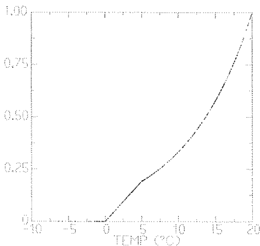
Figur 11.3. Mikroorganismernas relativa aktivitetsgrad (nedbrytning, nitrifikation och denitrifikation) i relation till marktemperaturen (TEMP). Från SOILN simulering av Blombäck & Eckersten (1997).
