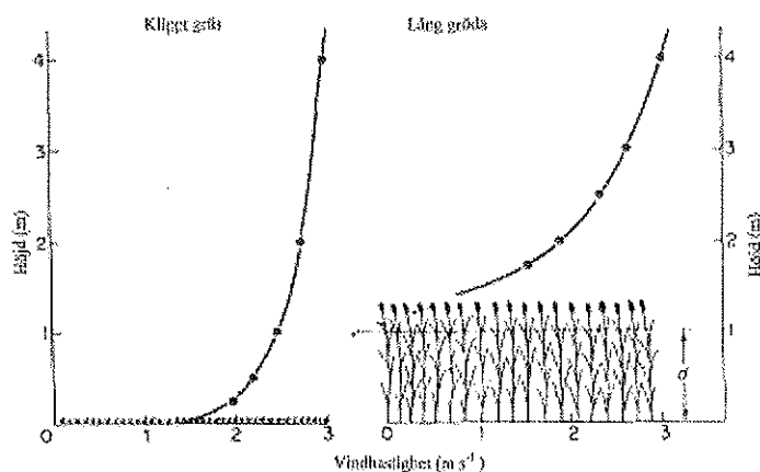
Fig 4.1 Vindprofil över ett lågt och jämnt respektive ett högt och ojämnt växttäck (Monteith & Unsworth 1990).
