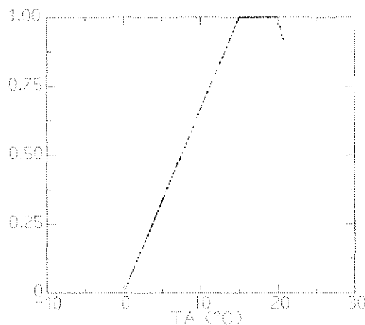
Figur 11.2. Kolupptagets (per dag) relativa respons på dygnsmedelvärdet av lufttemperaturen (TA). Från SOILN simulering av Blombäck & Eckersten (1997).
