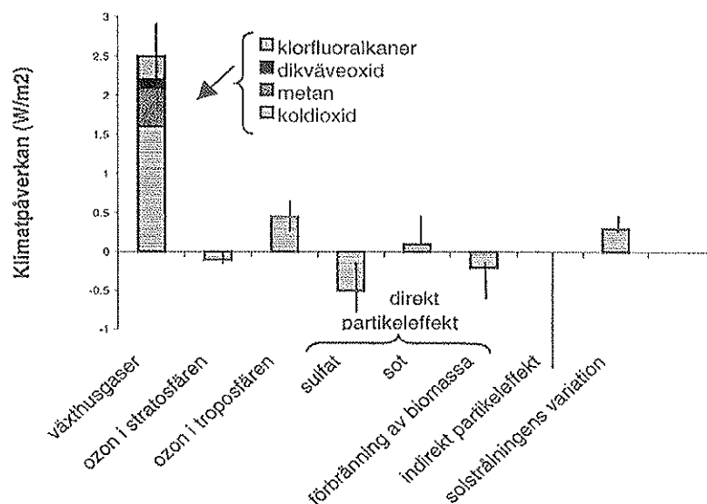
Figur 3.3. Jämförelse mellan olika faktorerers påverkan på det globala klimatet under de senaste hundra åren. Observera att ozon också är den växthusgas, trots att den inte ingår i stapeln med övriga växthusgaser. (Efter Rhode 1996).
