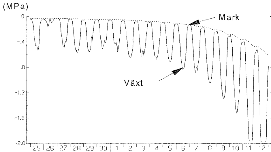
Figur 4.4a. Med SPAC-modellen simulerad vattenpotential i mark och växt under ett upptorkningsförlopp 25 juni till 12 juli 1994 i Uppsala. Växten är en energiskog (Salix) på en relativt lerig jord. Växtens vattenpotential sjunker kraftigt mitt på dagen men återhämtar sig på natten till markens vattenpotential, som dock sjunker successivt på grund av de ackumulerade vattenförlusterna genom avdunstning. Mot slutet av perioden blir vattenpotentialen i bladen så låg att bladen tenderar att vissna mitt på dagen.
