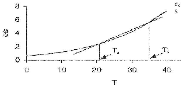
Figur 8.11. Grafisk beskrivning av s (ekv 8.28) som lutningen på mättnadsångtryck-temperaturkurvan vid medelvärdet av T_a och T_s .
