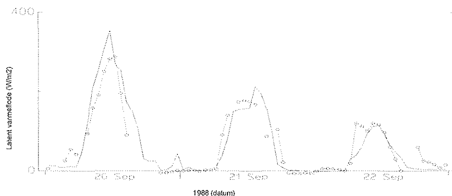
Figur 5.6. Simulerat (linje; SPAC-modellen) och mätt (punkter) latent värme flöde från ett Salixbestånd i Uppsala 20-22/9 1988. Regn föll på kvällen den 20/9. Mätningarna av vattenångeflödet och drivdata är gjorda av Anders Lindroth och medarbetare (SLU, Uppsala).
