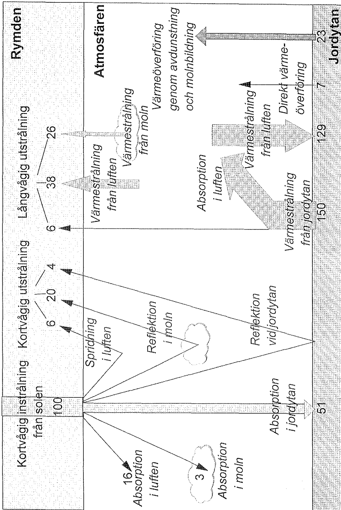
Figur 7.2. Jordens energibalans. (Omritad efter Sveriges Nationalatlas, 1995)
