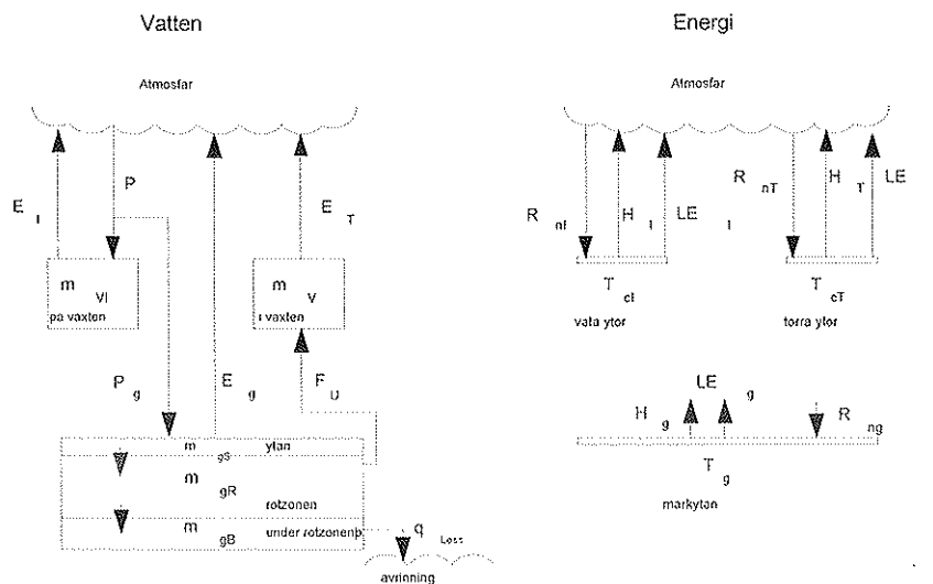
Figur 5.2. Schematisk beskrivning av SPAC modellen. Heldragna linjer är flöden av vatten och energi. För förklaring av symboler, se symbollista (Efter Eckersten 1995).
