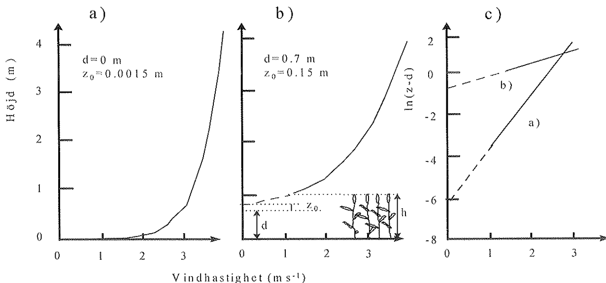
Figur 8.9. Tänkbara vindprofiler då vindhastigheten på 4 m är 3.5 \text{ ms}^{-1} för bar mark (a) och stråsäd (b) med motsvarande lin-log transformeringar (c). (Omritad efter Oke, 1978).
