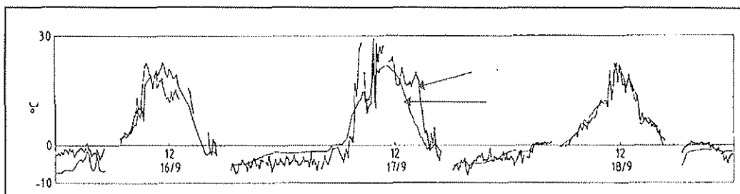
Figur 5.5. Simulerad (lång pil; SPAC-modellen) och mätt (kort pil) temperaturskillnad mellan blad och omgivande luft för ett Salixbestånd i Uppsala 16-18 september 1982 (Efter Eckersten 1986).
