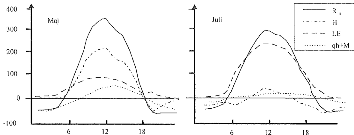
Figur 8.1. Exempel på dygnsfördelningen av komponenterna i energibalansen för ett energiskogsbestånd från två olika perioder under växstsäsongen ( PS mättades inte).
