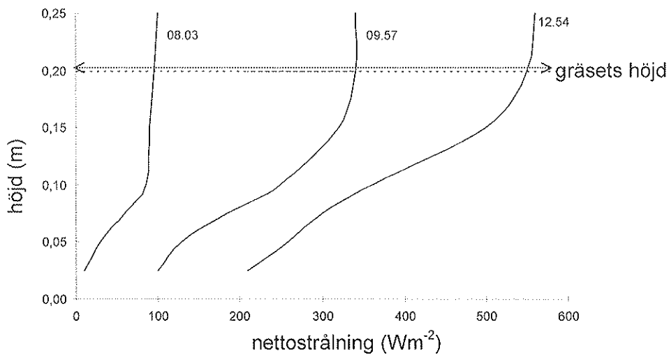
Figur 7.7. Nettostrålningen i ett 0,2 m högt gräsbestånd vid tre olika tidpunkter; 08.03, 09.57 och 12.54 (28 juni 1972, Saskatchewan). (Omritat efter Oke, 1978).
