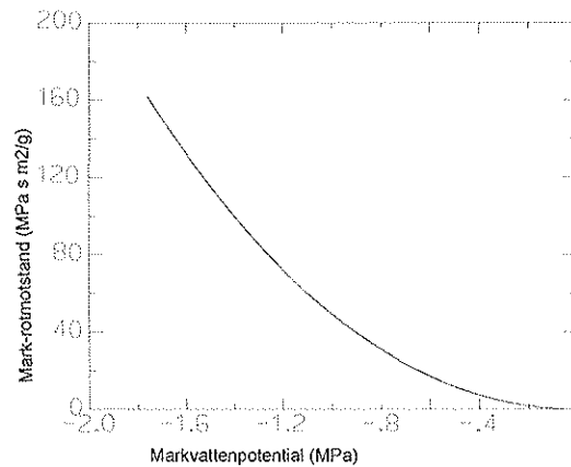
Figur 4.8. Mark-rotmotståndet r_g som funktion av markvattenpotentialen för samma jord som i figur 4.5a och b.
