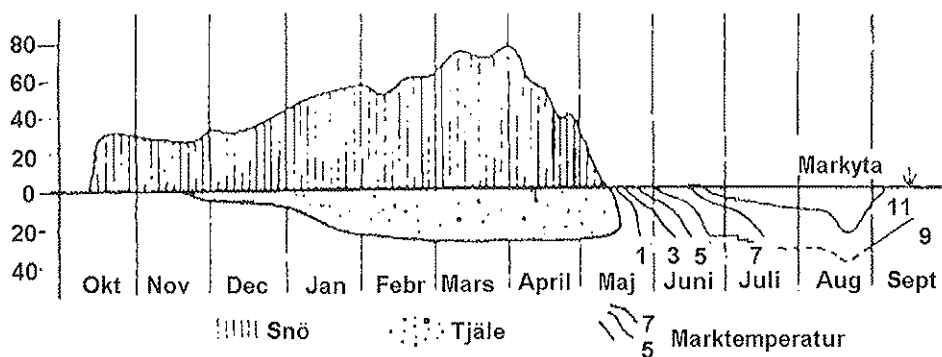
Figur 9.3. Tjäle och temperaturförhållanden i en tät granskog i Ångermanland. Översta figuren visar en ogallrad yta medan den undre visar förhållanden i motsvarande gallrad yta.
