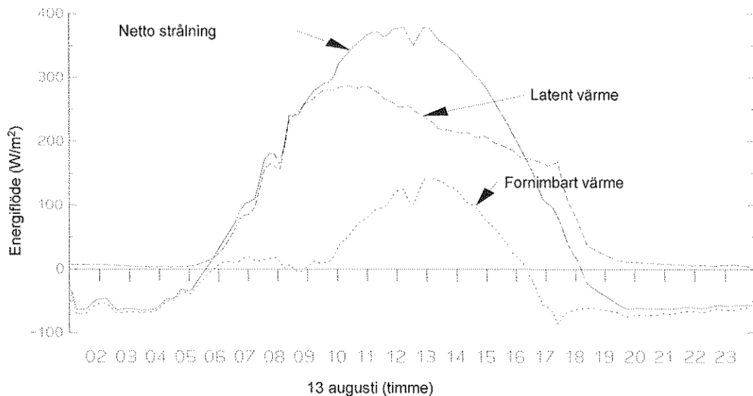
Figur 4.2. De olika komponenterna i bladens energibalans en solig sommardag i södra (mellersta Sverige. Nettostrålning som absorberats av lövverket = R_{nc} (baserad på mätningar), latent värme = LE_T , förnimbart (sensibelt) värme = H_T . Simuleringen av LE_T och H_T är gjord med SPAC modellen (se kap 5) för en Salixgröda med LAI = 5, på en mark med hög vattenpotential, i Uppsala 13 augusti 1989.
