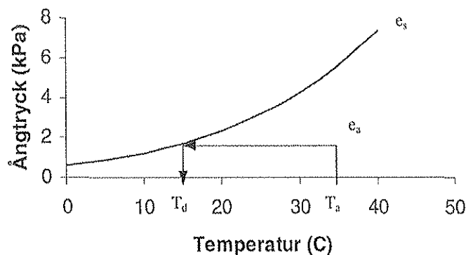
Figur 8.7. Schematisk bild över bestämning av daggpunktstemperatur. Vid en viss temperatur, T_a råder ett visst aktuellt ångtryck, e_a . Vid den punkt där e_a = e_s kan daggpunktstemperaturen, T_d , läsas av på x-axeln.
