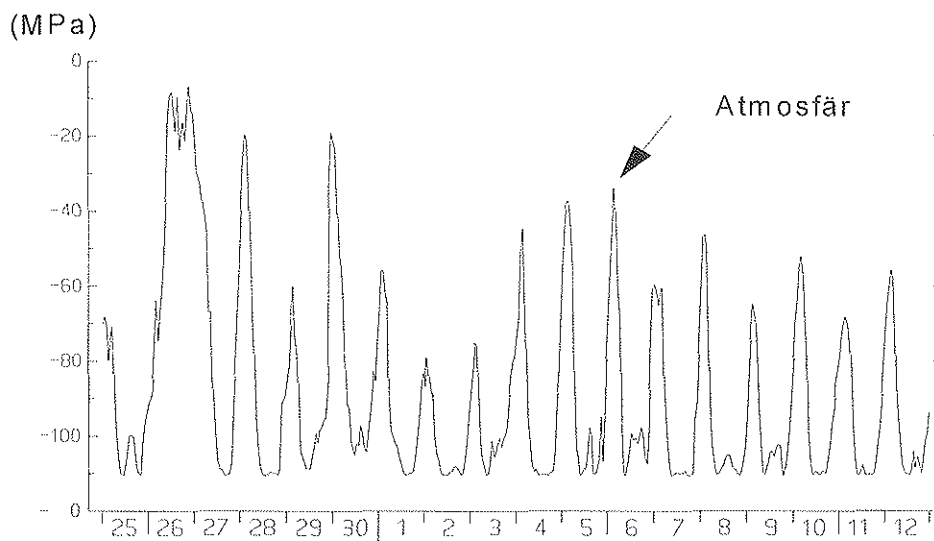
Figur 4.4b. Vattenpotentialen i atmosfären är oftast som lägst -10 MPa och på dagarna ca 100 ggr större än i mark och växt.
