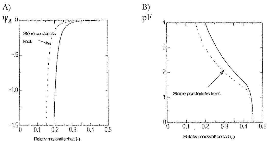
Figur 4.5. Markvattenpotentialen som en funktion av markens relativa vattenhalt.
