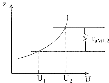
Figur 8.10. Schematisk bild över hur den aerodynamiska resistansen, r_{aM} beräknas utifrån vindhastigheten, U , på höjden z .
