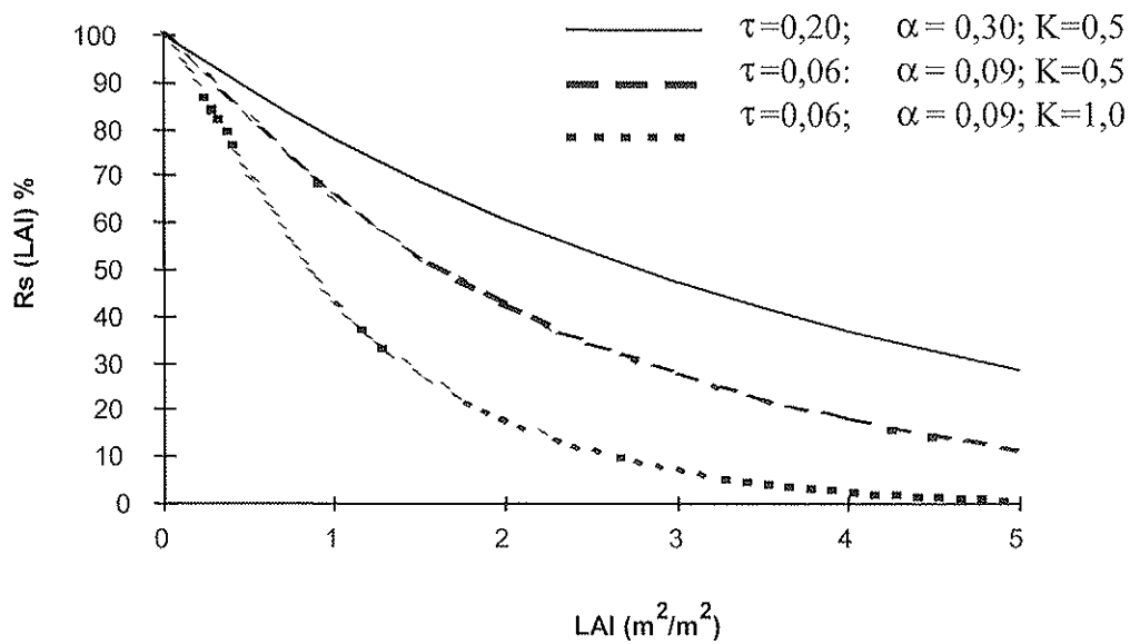
Figur 7.6. Det totala (dvs direkta + diffusa) flödet av kortvågig strålning i ett bestånd som funktion av bladyteindex LAI (räknat från bladverkets ovansida), beräknat enligt ekvation 7.15 och 7.16b. (a) Större delen av det kortvågiga spektrat (0,35-3,0 \mu\text{m} ), K=0,5 ; (b) PAR, K=0,5 ; (c) PAR, K=1 . (Omritat efter Torsell m fl 1989).
