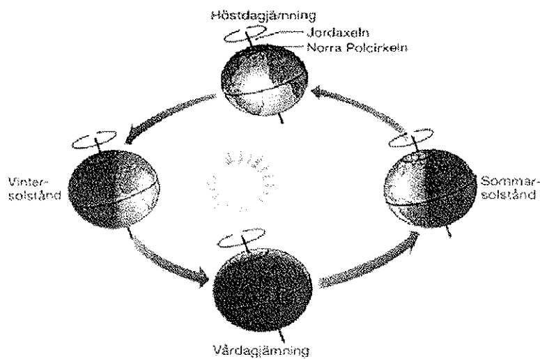
Figur 3.1 Jordklotets rörelse runt solen och sin egen axel. (SNA, 1995).
