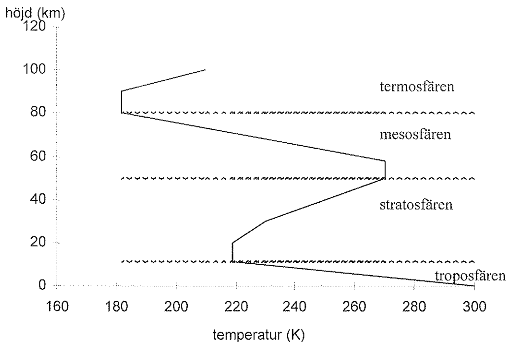
Figur 7.1. Atmosfärens vertikala indelning baserad på temperaturens variation med höjden. Underifrån räknat benämns skikten: Troposfären, stratosfären, mesosfären och termosfären. (Omritad efter Anomyn 1992).
