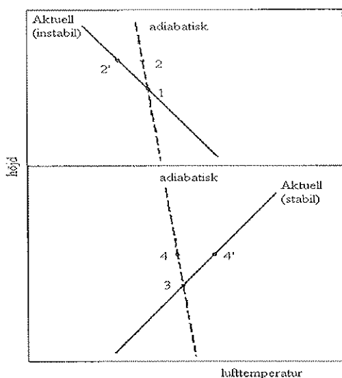
Figur 8.4. Schematisk bild av aktuell och adiabatisk temperaturprofil, vilka illustrerar termiskt instabila respektive stabila förhållanden i atmosfären. (Omritat efter Rosenberg et al, 1983).
