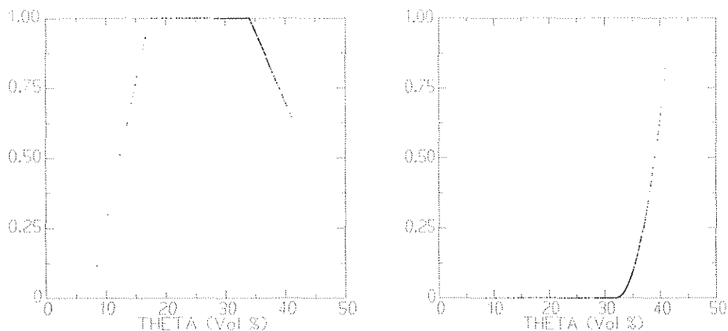
Figur 11.4 a) Aeroba mikroorganismers relativa aktivitetsgrad (nedbrytning och nitrifikation) i relation till markvattenhalten (THETA). b) Anaeroba mikroorganismers relativa aktivitetsgrad (denitrifikation) i relation till markvattenhalten. Från SOILN simulering av Blombäck & Eckersten (1997).
