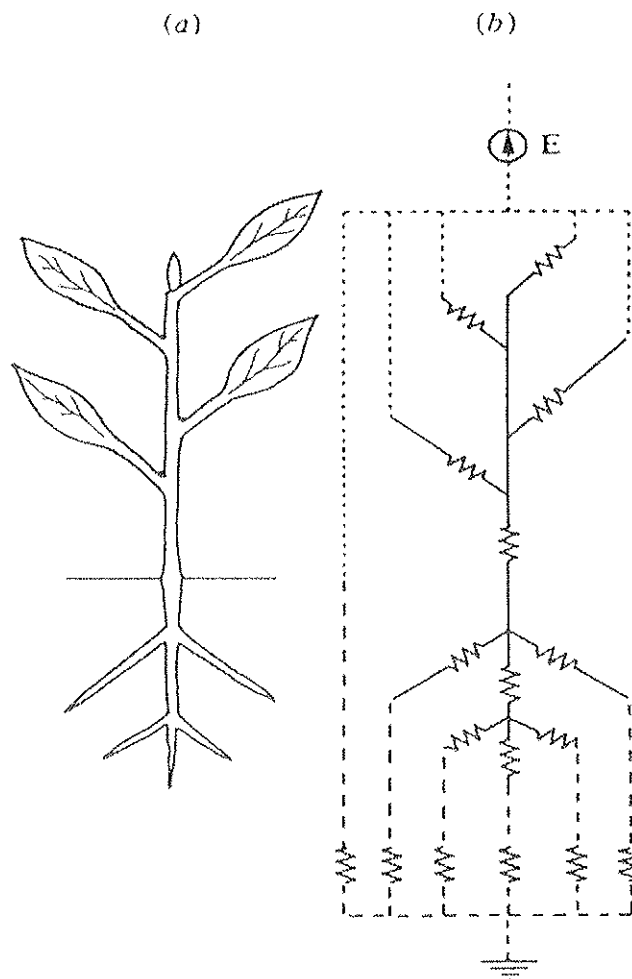
Figur 6.3 (a) Förenklad skiss av en växt; (b) Korresponderande flödesmotstånd i mark, rötter, stam och blad (Jones 1992).
