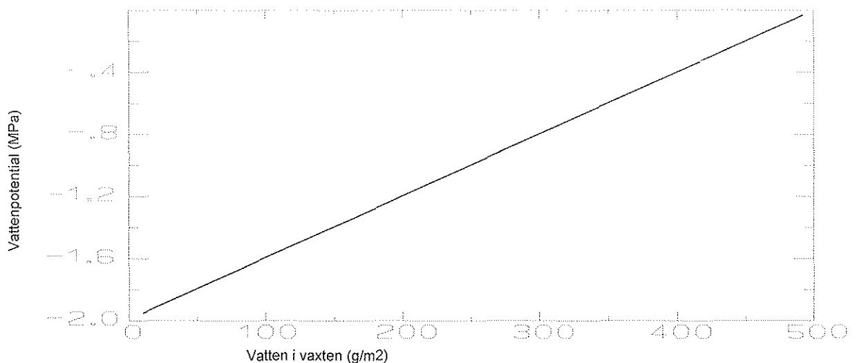
Figur 4.6. Bladens vattenpotential som funktion av växtens innehåll av lättillgängligt vatten. \Psi_c = \Psi_{cMax} = (\Psi_{cMax} - \Psi_{cMin})(1 - m_V / m_{VMax}) . Relationen har använts i simuleringarna presenterade i figur 4.1-4.4, 4.8-4.10 och 5.1.
