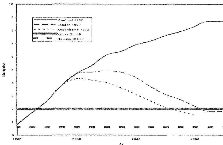
Figur 3.4. Uppmätt klorhalt i stratosfären sedan 1960, samt modellberäknade prognoser för framtiden enligt olika avvecklingsstrategier. (Efter Janson och Lejenäs, 1992)
