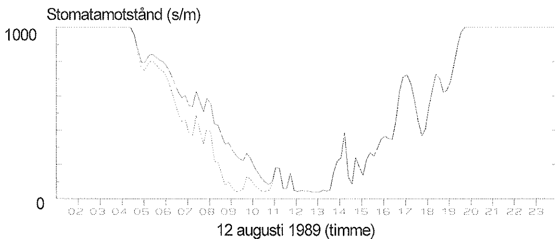
Figur 4.11. Stomatamotståndet uttryckt per markyttenhet, d v s sammantaget för hela lövverket, för en regnig dag, det faktiska motståndet (heldragen linje) och det motstånd som skulle varit om alla bladytor vore torra (samma förutsättningar som i figur 4.9).
