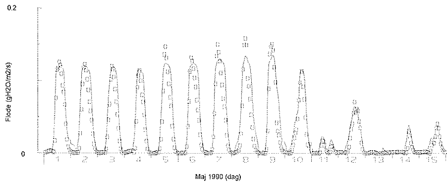
Figur 5.7. Simulerat (linje; SPAC-modellen) och mätt (punkter) vattenupptag för två 25-åriga granar i Skogaby (Halland) (Data efter Cienciala m fl 1994).
