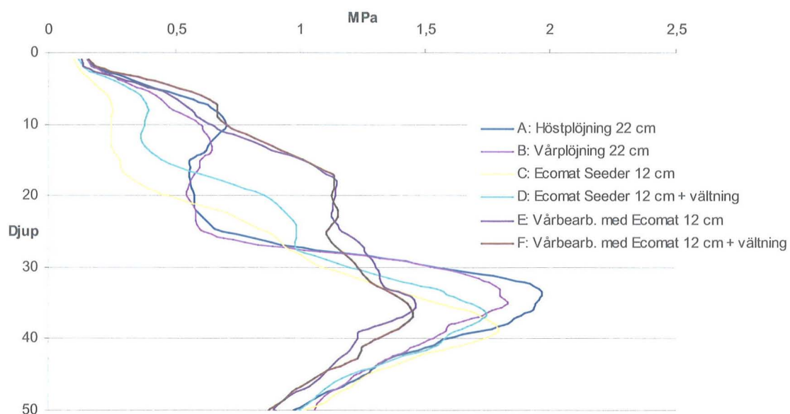
Figur 4 Penetromettermätningar nr 662, 30 % ler.
