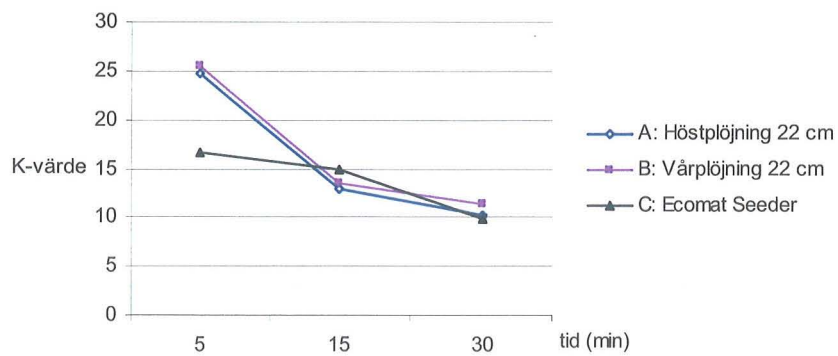
Figur 8. Infiltrationshastighet i försök nr 662.
