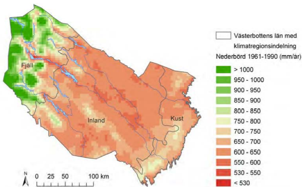
Figure 17. Annual average precipitation for Vasterbottens Lan for normal period 1961-1990. (Årsmedelnederbörd under referensperioden 1961 – 1990) (from Länsstyrelsen Västerbotten 2011).
