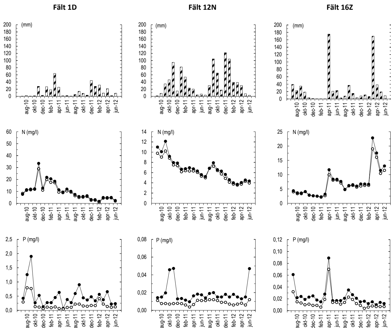
Figur 8. Månadsvis avrinning, flödesvägda månadsmedelhalter av totalkväve (●) och nitratkväve (○), samt av totalfosfor (●) och fosfatfosfor (○) perioden juli 2010 till juni 2012 på fält 1D, 12N och 16Z. Observera olika skalor på y-axlarna.
