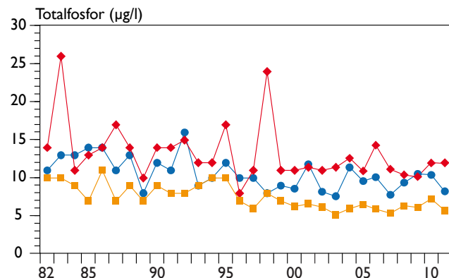
Figur 5. Totalfosforhalt i ytvatten (0,5 m) vid M1 och M2 i Mariestadsfjärden, samt vid Dagskärsgrund i Storvänern. Samtliga data är medelvärden för resp. provtagningsår 1982–2011. Symboler enligt figur 3.
