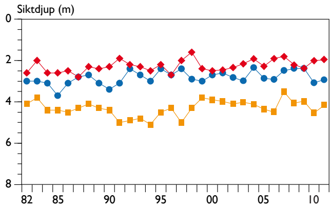
Figur 7. Siktdjupet vid M1 och M2 i Mariestadsfjärden, samt Dagskärsgrund i Storvänern. Samtliga data är medelvärden för resp. provtagningssäsong 1982–2011. Symboler enligt figur 3.
