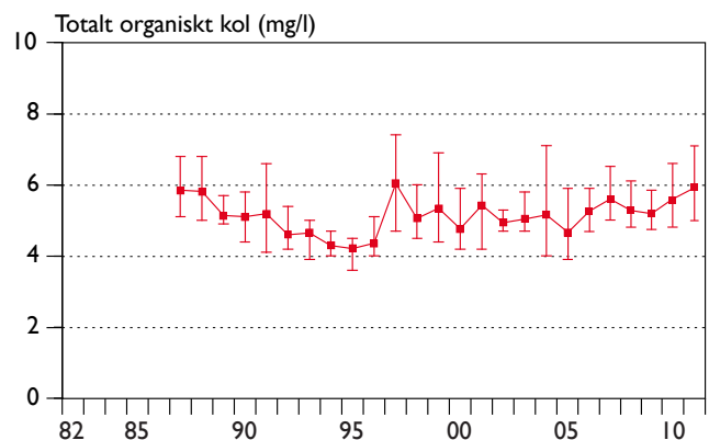
Figur 10. Mängden organiskt material (uttryckt som TOC) i Mariestadsfjärdens ytvatten (0,5 m) vid station M2 1986–2011. Medel-, min- och max-värden anges för respektive säsong.
