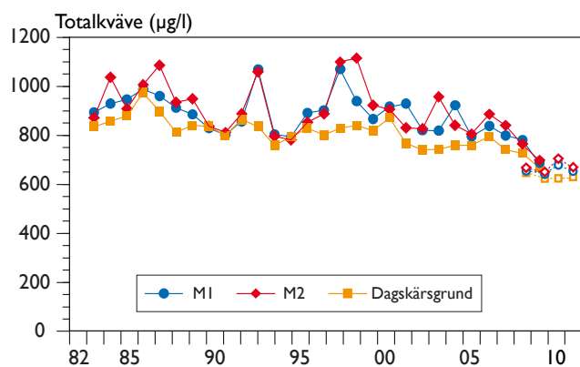
Figur 3. Totalkvävehalt i ytvatten (0,5 m) vid M1 och M2 i Mariestadsfjärden, samt vid Dagskärsgrund i Storvänern. Samtliga data är medelvärden för resp. provtagningsår 1982–2011. Analysmetoden för totalkväve har ändrats och sker fr o m 2010 enbart med den s k TNb-metoden (ihåliga markeringar och streckade linjer), från att fram till och med 2009 ha skett med den s k summa-metoden (homogena markeringar och linjer).
