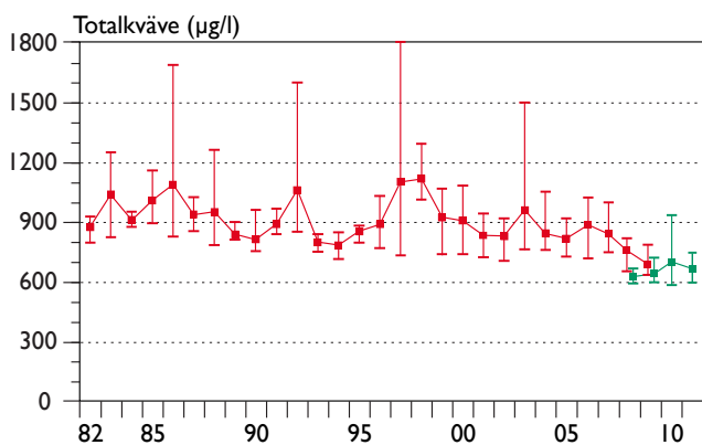
Figur 2. Totalkvävehalt i Mariestadsfjärdens ytvatten (0,5 m) vid station M2 1982–2011. Medel-, min- och maxvärden anges för resp. provtagningsår. Analysmetoden för totalkväve har ändrats och sker fr o m 2010 enbart med den s k TNb-metoden (grönt), från att fram till och med 2009 ha skett med den s k summa-metoden (rött).
