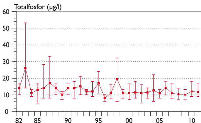
Figur 4. Totalfosforhalt i Mariestadsfjärdens ytvatten (0,5 m) vid station M2 1982–2011. Medel-, min- och maxvärden anges för resp. provtagningsår.
