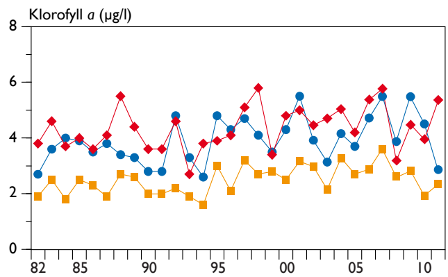
Figur 9. Klorofyllhalt i ytvatten (0,5 m) vid M1 och M2 i Mariestadsfjärden, samt vid Dagskärsgrund i Storvänern. Samtliga data är medelvärden för resp. provtagningssäsong 1982–2011. Symboler enligt figur 3.
