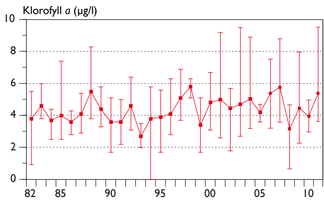
Figur 8. Klorofyllhalt i Mariestadsfjärdens ytvatten (0,5 m) vid station M2 1982–2011. Medel-, min- och maxvärden anges för resp. provtagningssäsong.
