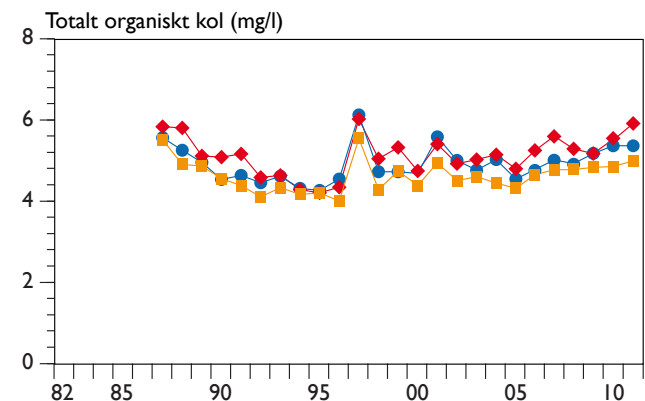
Figur 11. Mängden organiskt material (uttryckt som TOC) i ytvatten (0,5 m) vid M1 och M2 i Mariestadsfjärden, samt Dagskärsgrund i Storvänern. Medelvärden för resp. provtagningssäsong 1986–2011. Symboler enligt figur 3.
