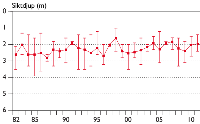
Figur 6. Siktdjupet i Mariestadsfjärden vid station M2 1982–2011. Medel-, min- och max-värden anges för resp. provtagningssäsong.
