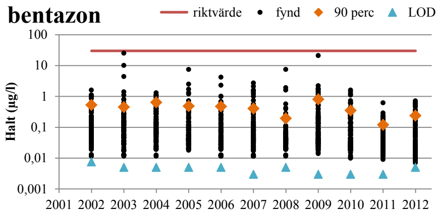
Figur 47. Fynd av bentazon i de fyra typområdena och åarna, per år, jämfört med riktvärdet (röd linje). Orange symbol (90 perc) anger vid vilken nivå 90% av proverna hade en lägre halt (eller ingen uppmätt halt alls) respektive år. Blå symbol anger detektionsgränsen (LOD; medianvärde) respektive år.
