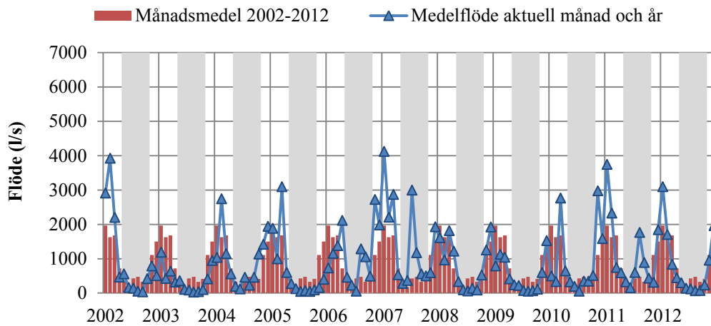
Figur B1 – 13. Vattenflöde (l/s) i Skivarsån, medelflöde per månad 2002-2012 jämfört med månadsmedel för samma period. Grå bakgrund indikerar maj till och med oktober, dvs ordinarie provtagningsperiod för ytvatten.
