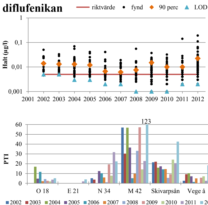
Figur 49. Övre figuren visar fynd av diflufenikan i de fyra typområdena och åarna, per år, jämfört med riktvärdet (röd linje). Orange symbol (90 perc) anger vid vilken nivå 90% av proverna hade en lägre halt (eller ingen uppmätt halt alls) respektive år. Blå symbol anger detektionsgränsen (LOD; medianvärde) respektive år. Undre figuren visar PTI (toxicitetsindex som visar storleken på riktvärdesöverskridandet) per år och område där O18: Västergötland; E21 Östergötland; N34: Halland; M42: Skåne.
