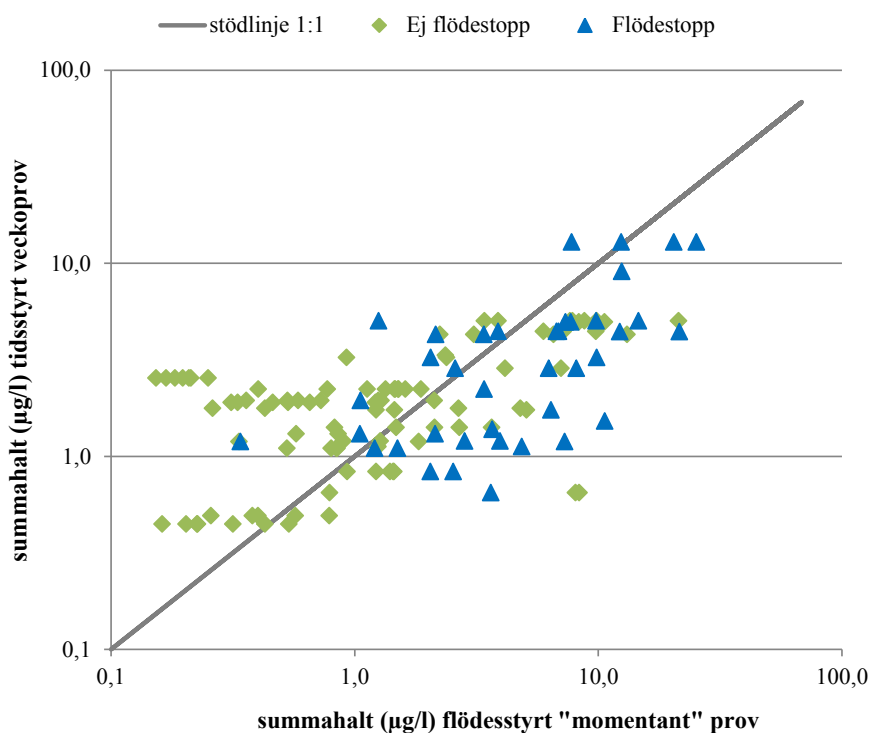
Figur 41. Summahalten i prov taget med flödesstyrd provtagare jämfört med summahalten i ett tidsstyrt prov taget under motsvarande (samma) vecka. Blå (trekant) och grön (fyrkant) visar om flödesprovet togs under en flödestopp eller inte (ej flödestopp, d.v.s. innan eller efter en topp). I vissa fall har flera flödesstyrda prover tagit under en och samma vecka. Figuren innehåller 135 utav 143 insamlade flödesstyrda prover då en vecka saknade motsvarande tidsstyrt veckoprov. Flödesproverna kan betraktas som momentanprov, bortsett från 2012 års prover som består av tre delprov tagna under kort tid, därav citationstecken kring momentan.
