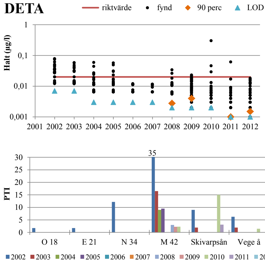
Figur 62. Övre figuren visar fynd av DETA (terbutylazindesetyl) i de fyra typområdena och åarna, per år, jämfört med riktvärdet (röd linje). Orange symbol (90 perc) anger vid vilken nivå 90% av proverna hade en lägre halt (eller ingen uppmätt halt alls) respektive år. Blå symbol anger detektionsgränsen (LOD; medianvärde) respektive år. Undre figuren visar PTI (toxicitetsindex som visar storleken på riktvärdesöverskridandet) per år och område där O18: Västergötland; E21 Östergötland; N34: Halland; M42: Skåne.
