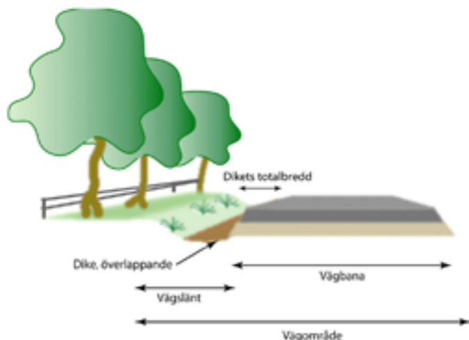
Figur 8.4: Exempel på olika vegetationsremsor, och hur de kan ansluta till andra linjeobjekt. Dikesrenar och väglänter kan både ansluta och överlappa med diken.
