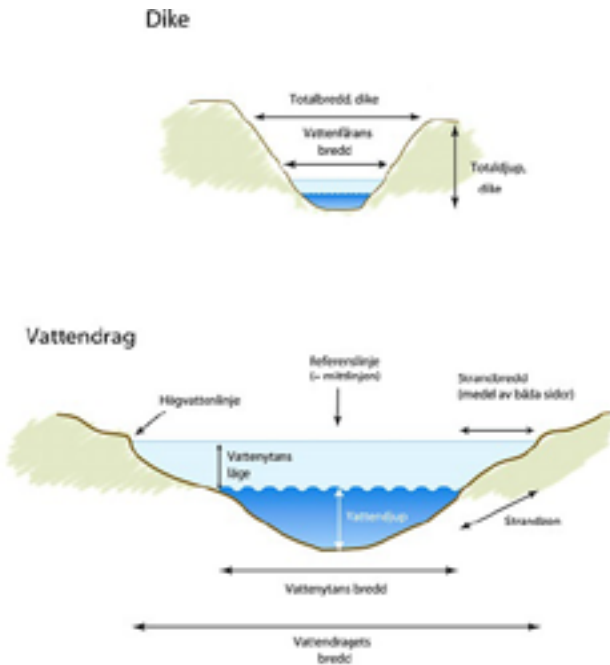
Figur 8.7. Beskrivning av referenslinjer och beskrivna zoner i diken och vattendrag.
