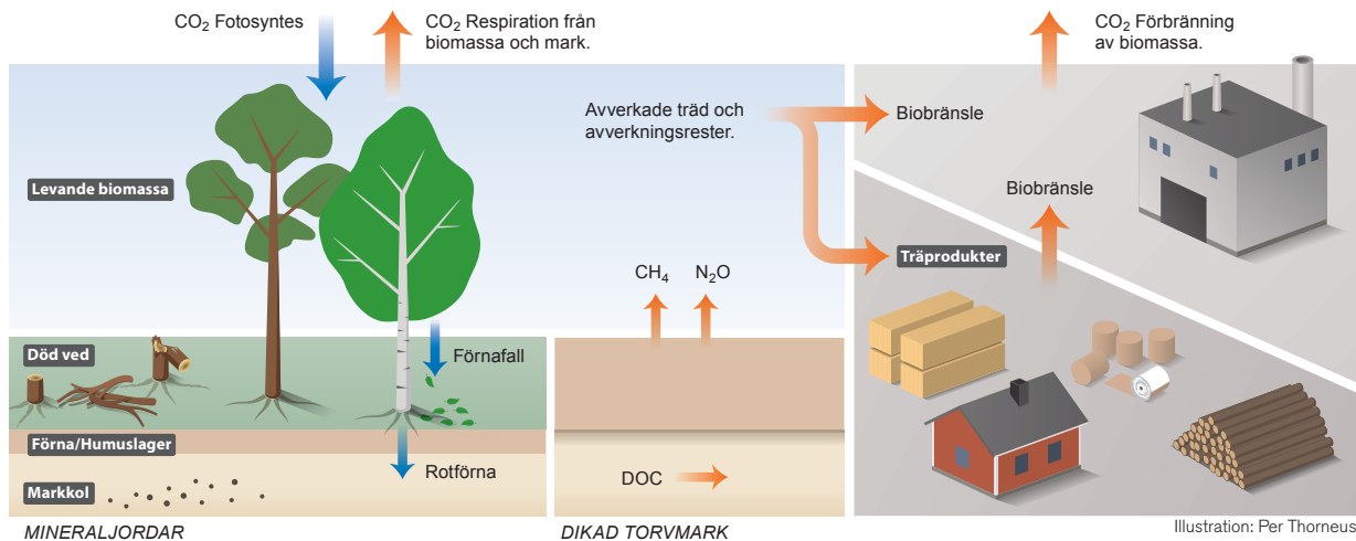
Figur 2. Figuren visar kolets kretslopp i förhållande till de kolpooler (vit text med grå bakgrund) som redovisas i klimatrapporteringen. Kolförrädsförändringar som rapporteras representerar skillnaden mellan inflödet och utflödet av kol för en kolpool. För kolpoolen levande biomassa representerar kolförrädsförändringen skillnaden mellan upptag genom fotosyntes och utsläpp på grund av respiration, avverkning och naturlig avgång.
